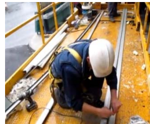
Corte guía inferior
