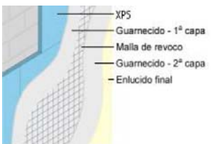
XPS y acabado en yeso
